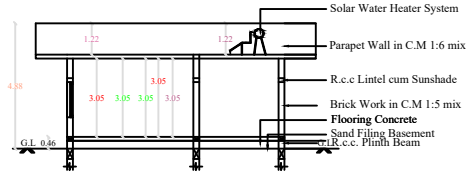
SECTION A-B
