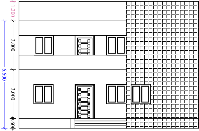
ELEVATION
