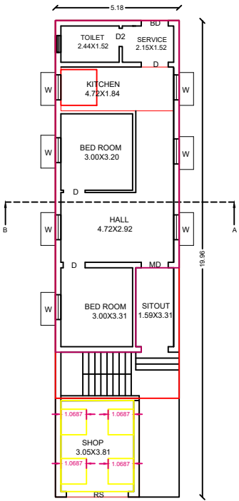
UND FLOOR PLAN
