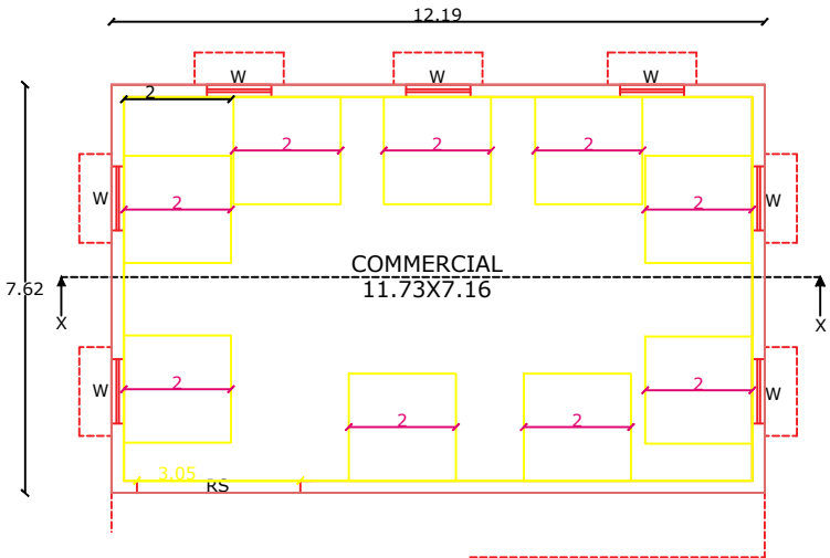
DOOR PLAN
