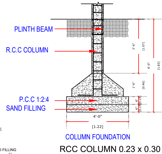
RCC COLUMN 0.23 x 0.30
