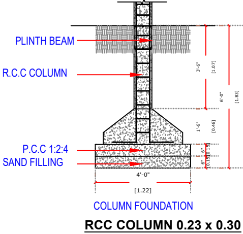
RCC COLUMN 0.23 x 0.30
