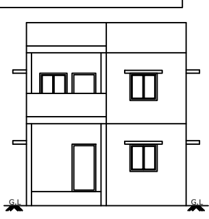
ELEVATION
