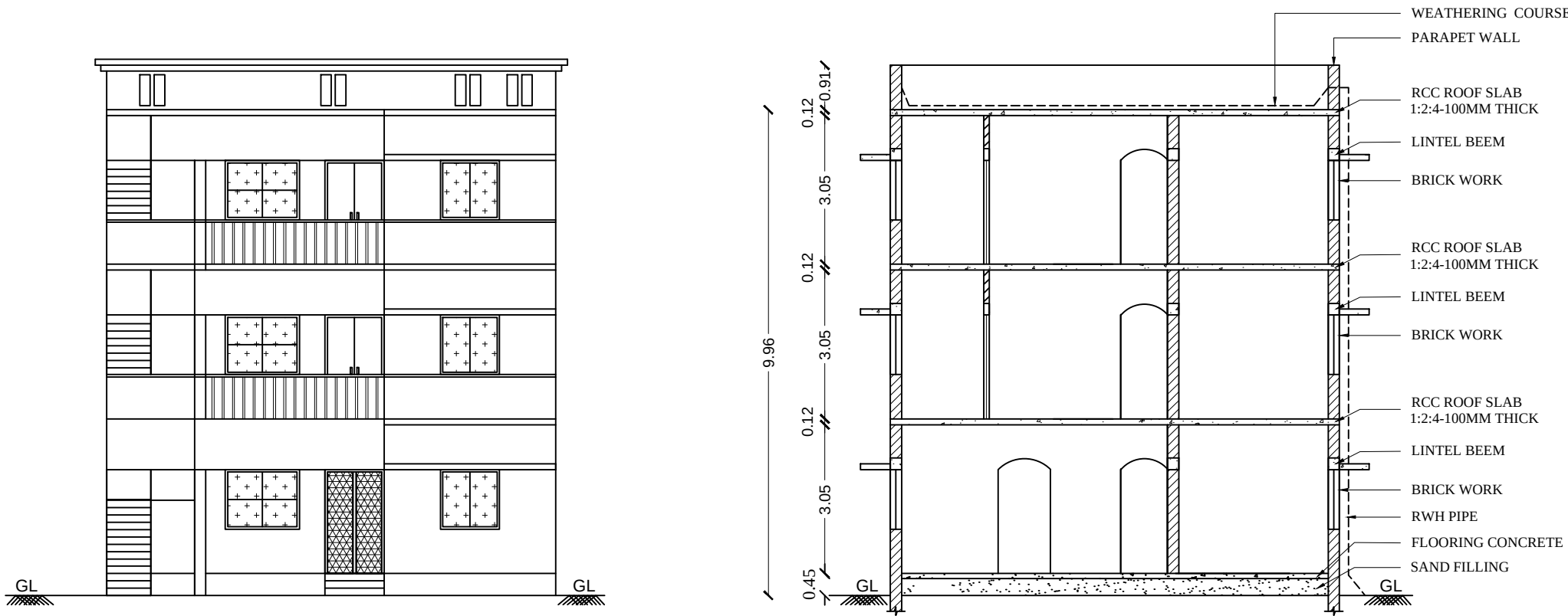
ELEVATION
