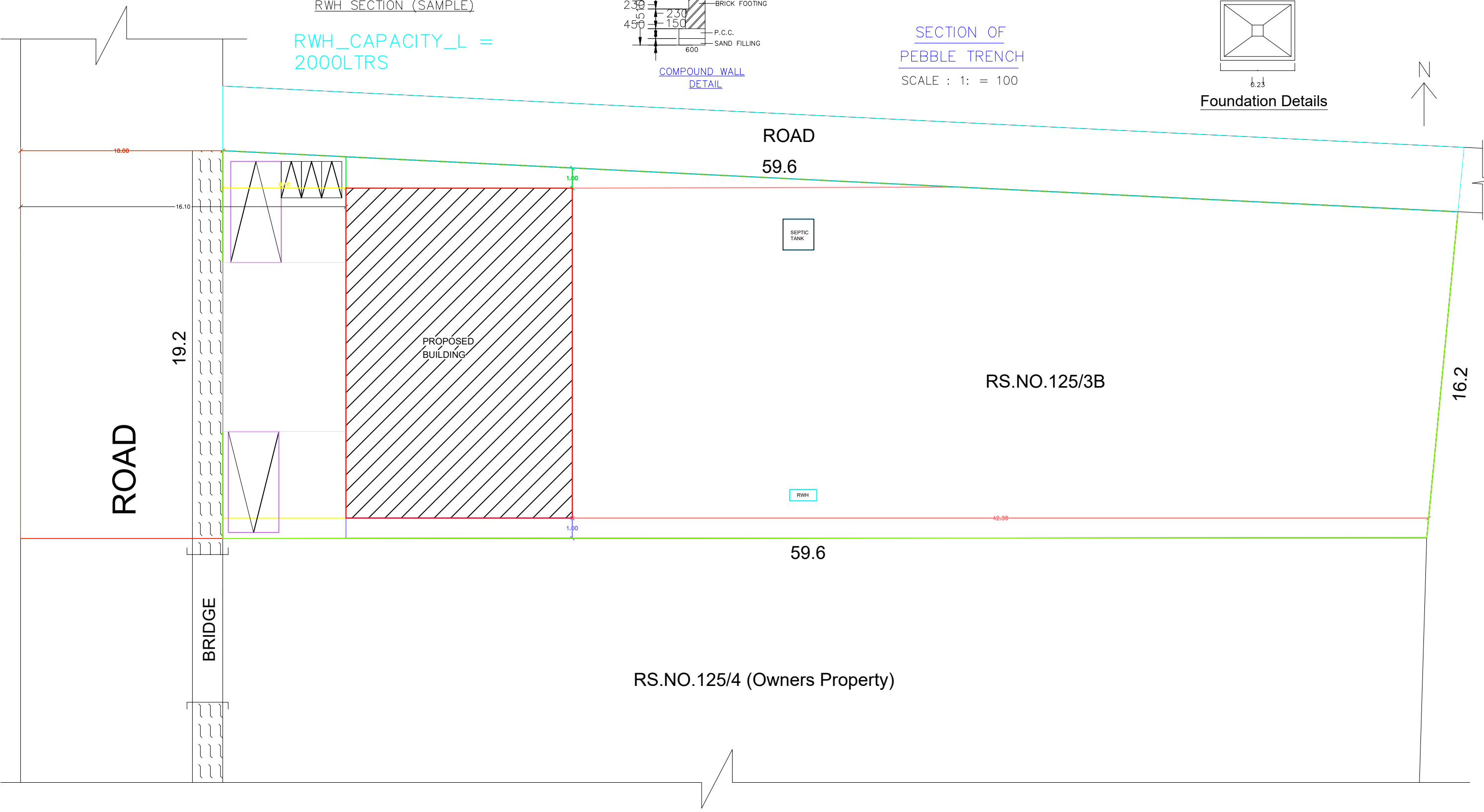
SITE PLAN-1:100
