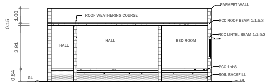
SECTION A-B
