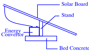
LONGITUDINAL SECTION
