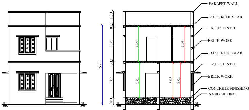
ELEVATION
