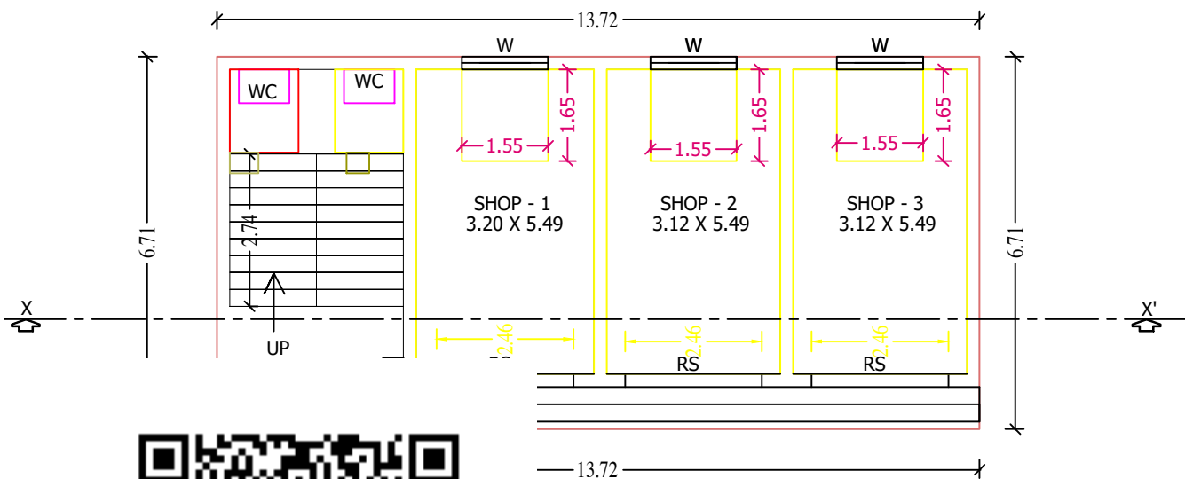
UND FLOOR PLAN
