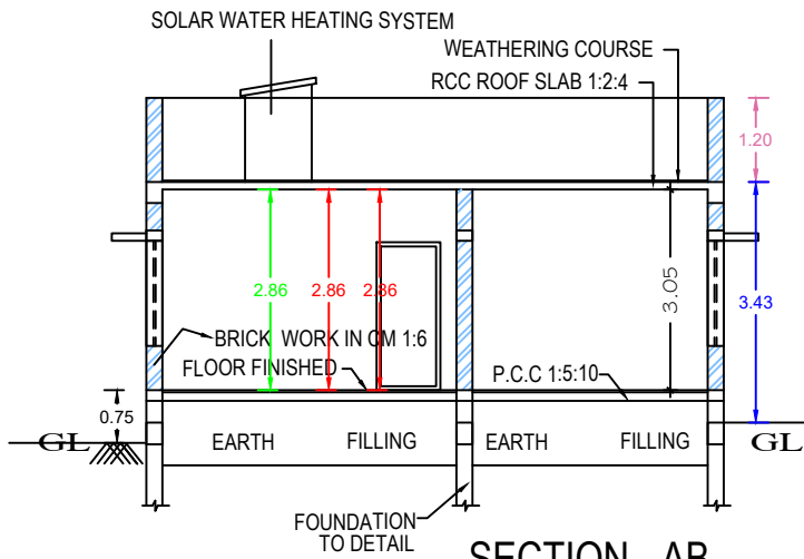
SECTION - AB
