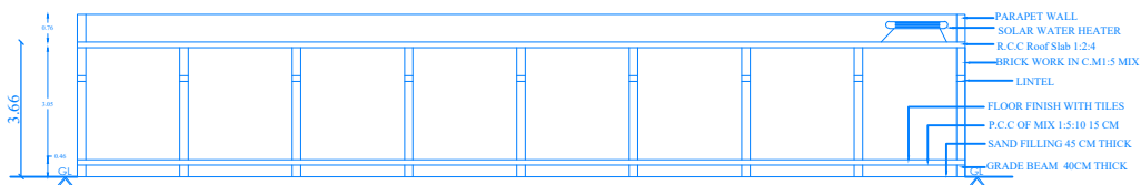
SECTION A-A
