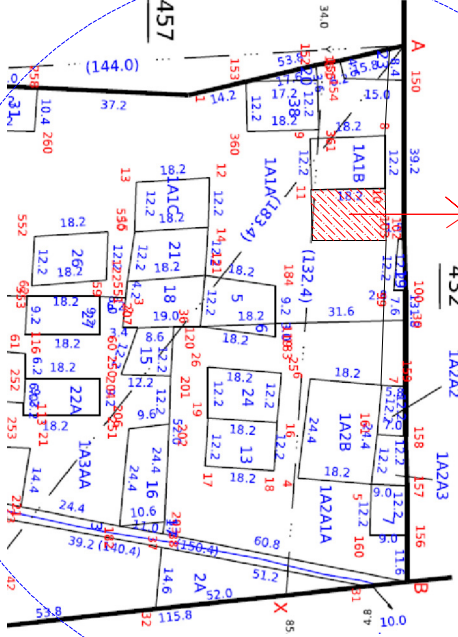
Key Plan - Scale 1 : 500 )
