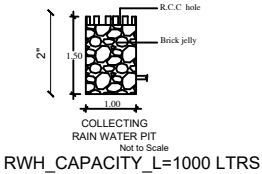
RWH_CAPACITY_L=1000 LTRS
