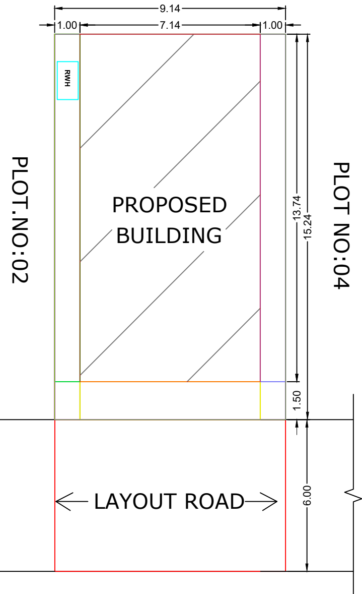
SITE PLAN: 1:100
