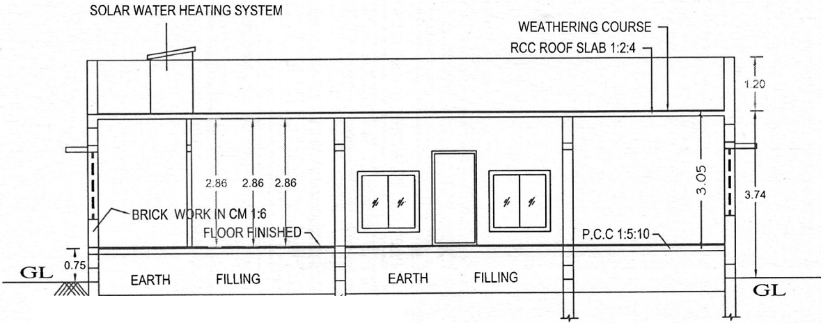
SECTION - AB
