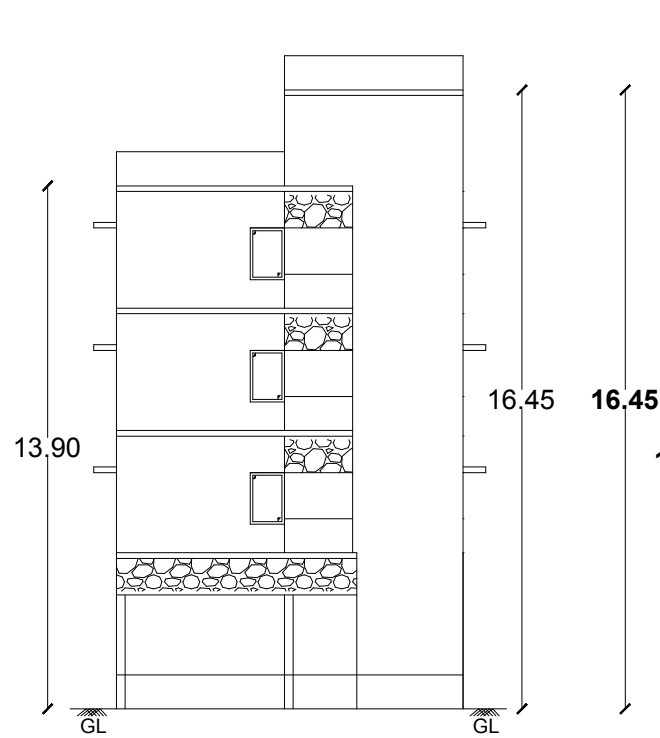
ELEVATION
