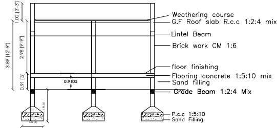
SECTION A-B
