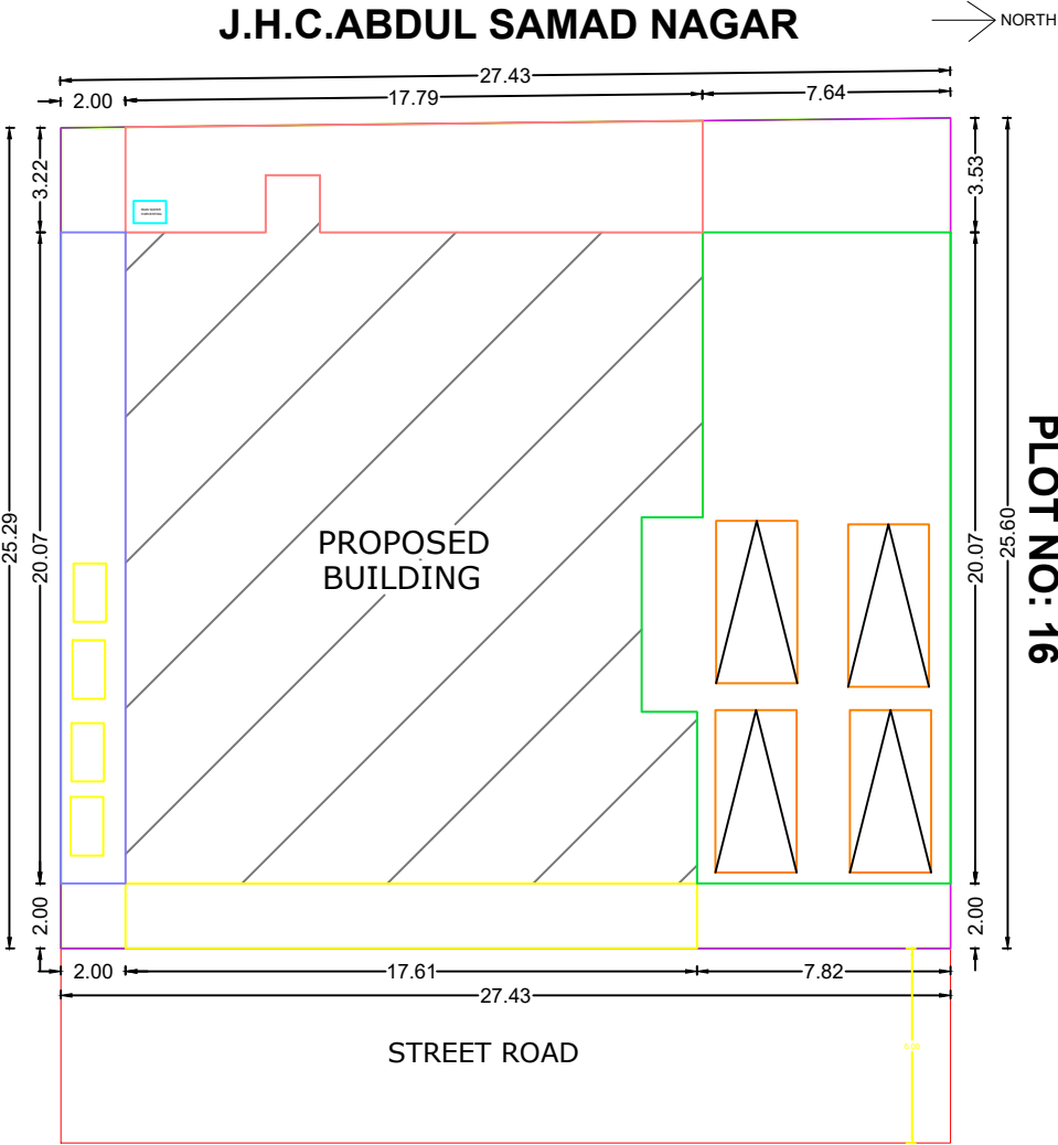
SITE PLAN: 1:100
