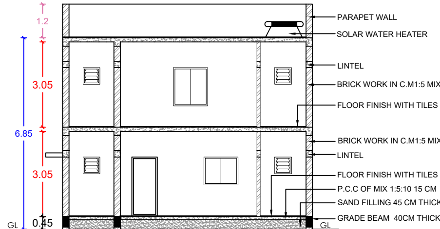
SECTION A-B
