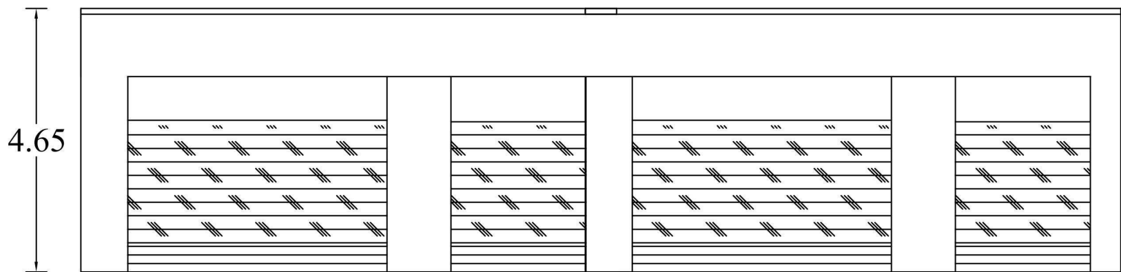
ELEVATION
