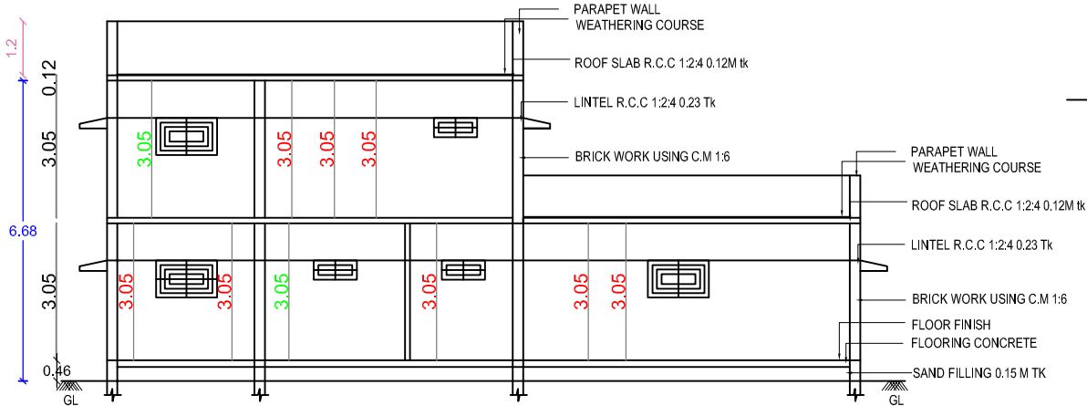
SECTION A-B
