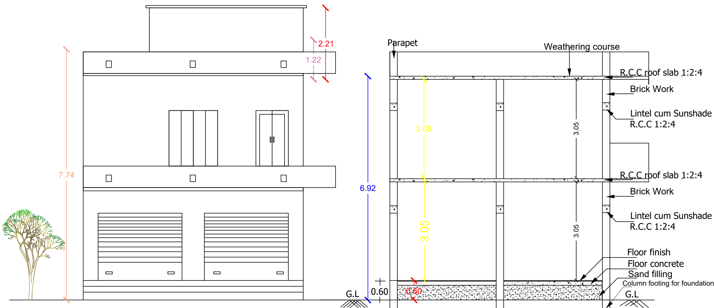
ELEVATION
