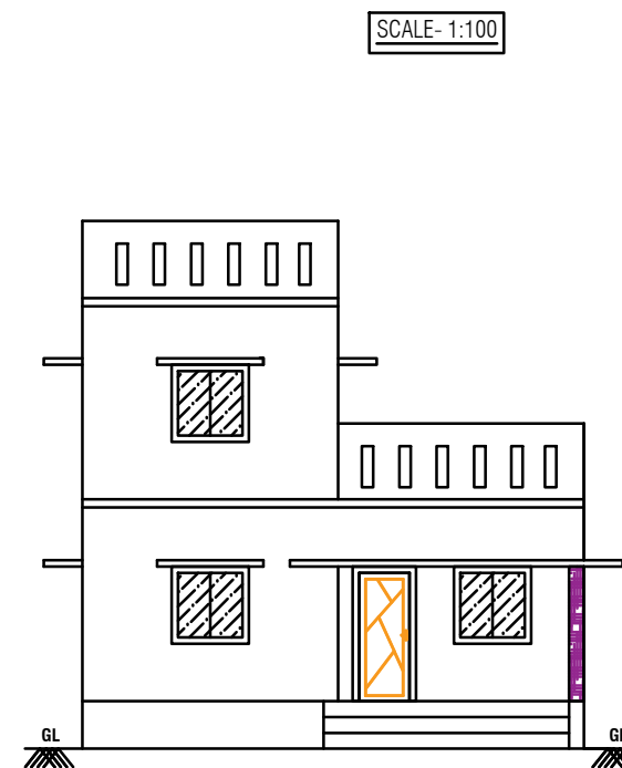
ELEVATION 7.92
