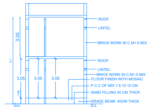
SECTION -AB
