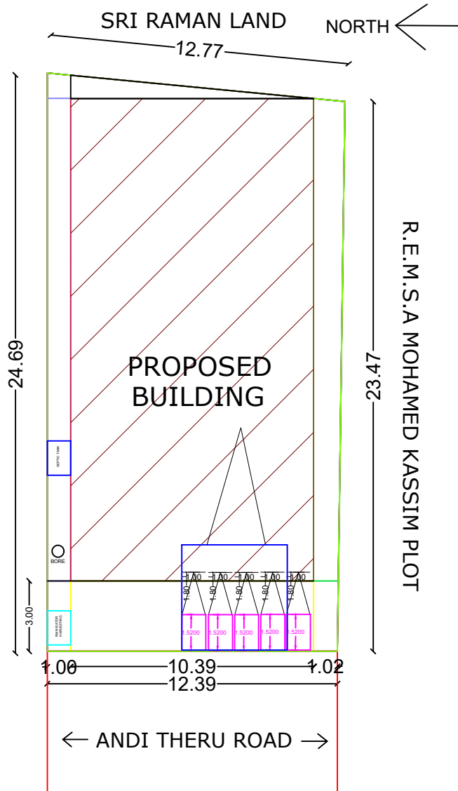
SITE PLAN: 1:100
