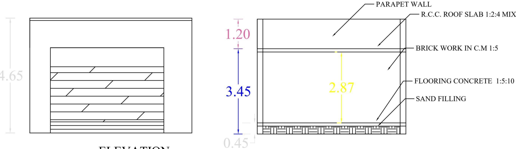
ELEVATION
