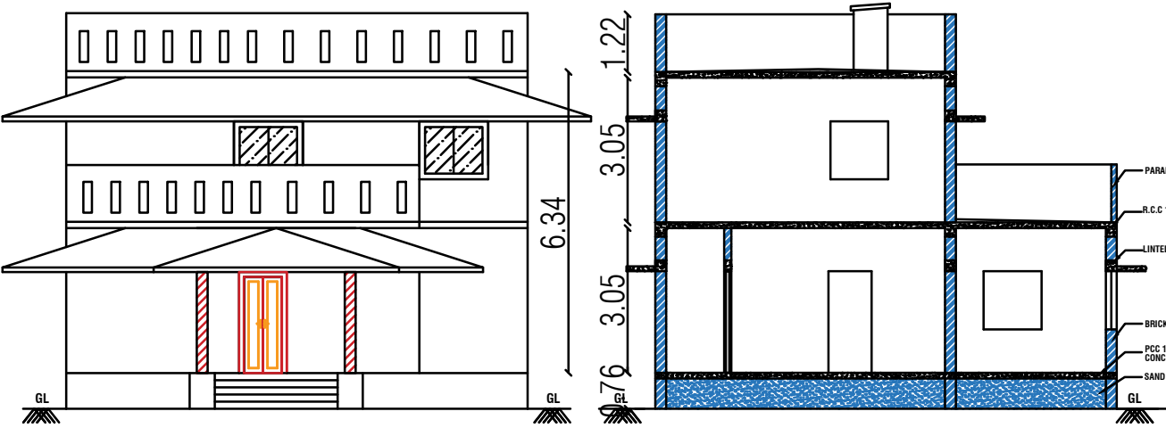
ELEVATION
