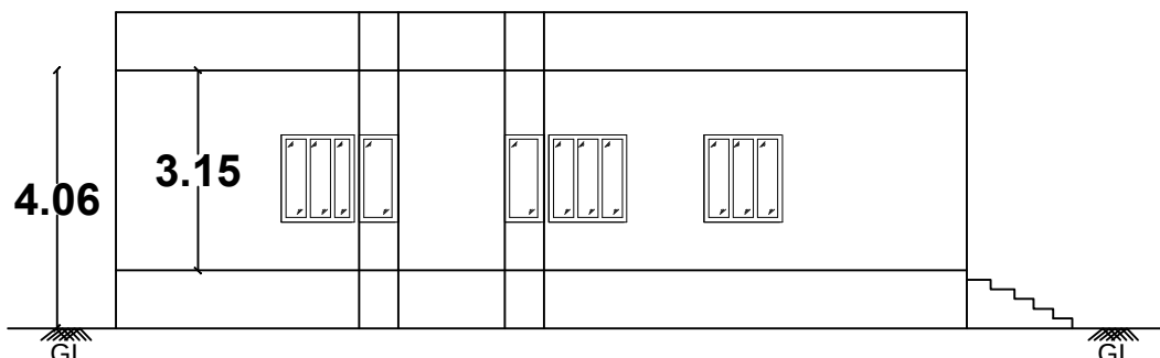
ELEVATION
