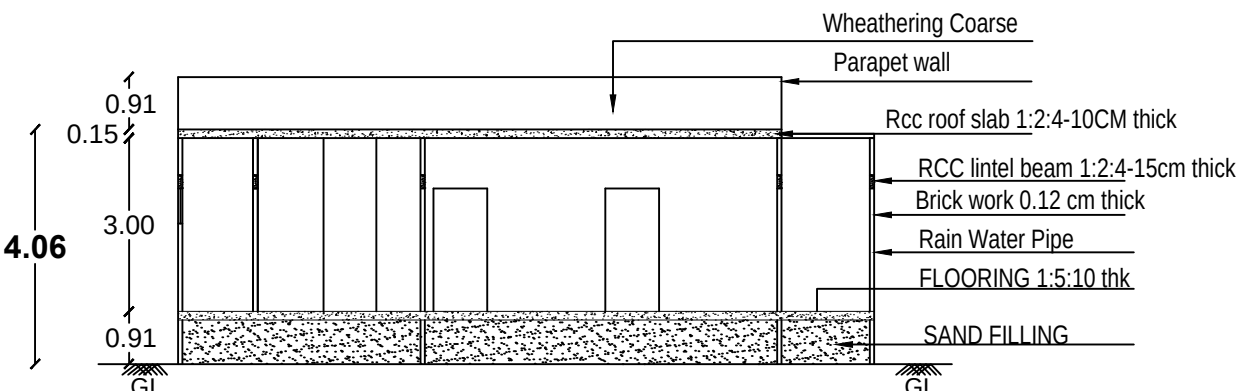
SECTION - AB
