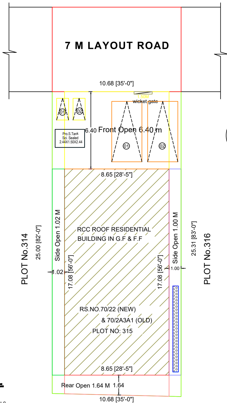
NANJAI LAND SITE PLAN
