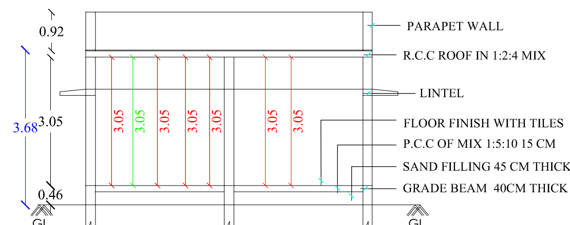
SECTION A-B
