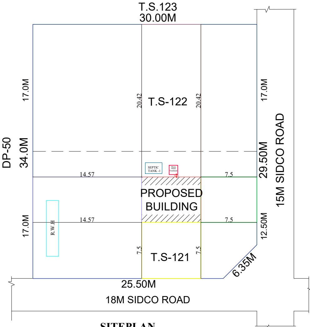
SITEPLAN 1:200
