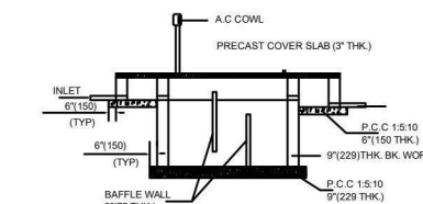
SECTION XX- XX
