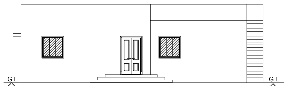
ELEVATION
