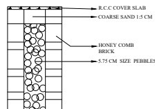
0.20.30.23 SECTION
