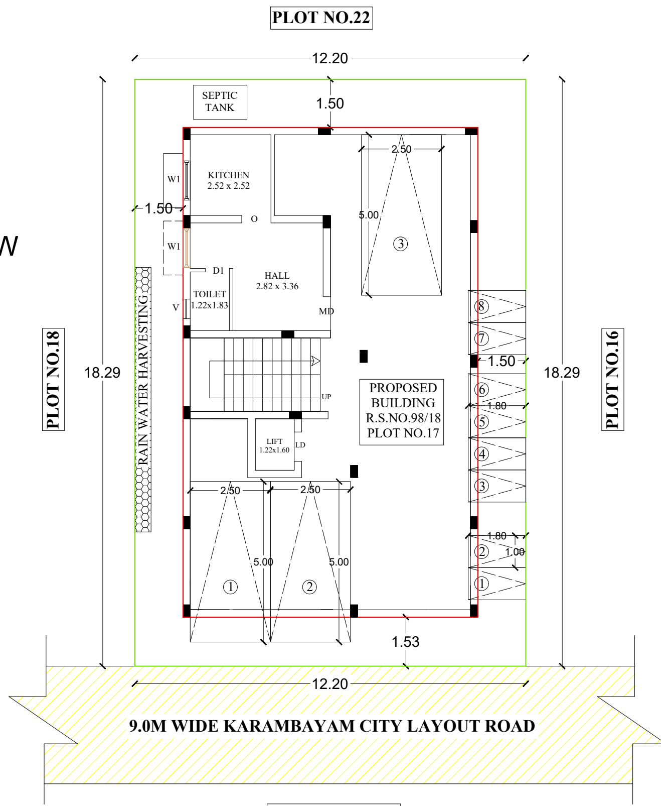
SITEPLAN SCALE : 1: 100
