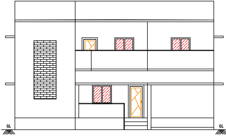
ELEVATION
