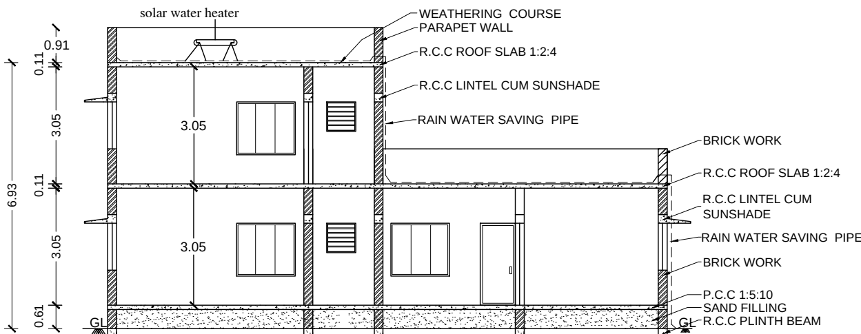
SECTION 'AB'
