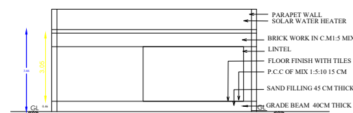
SECTION -AB
