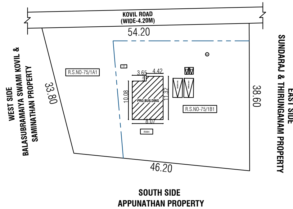
SITE PLAN SCALE - 1:400
