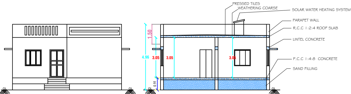
ELEVATION
