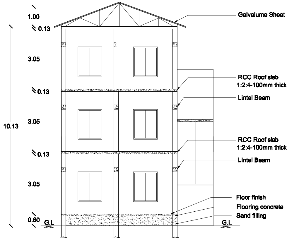
SECTION ON DE
