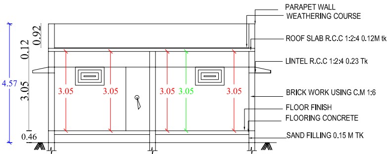
SECTION A-B
