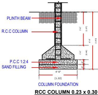
RCC COLUMN 0.23 x 0.30
