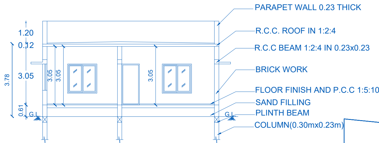
SECTION A-B
