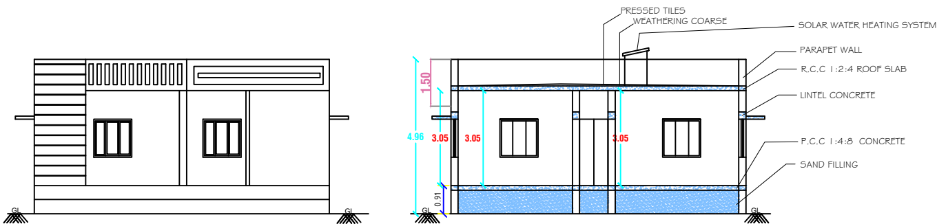
ELEVATION
