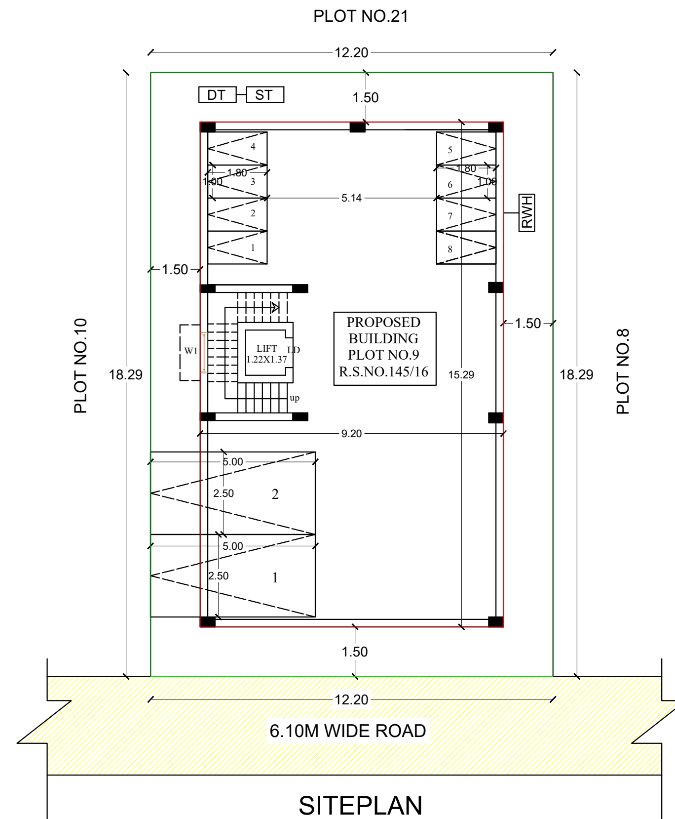
SITEPLAN SCALE : 1: 100
